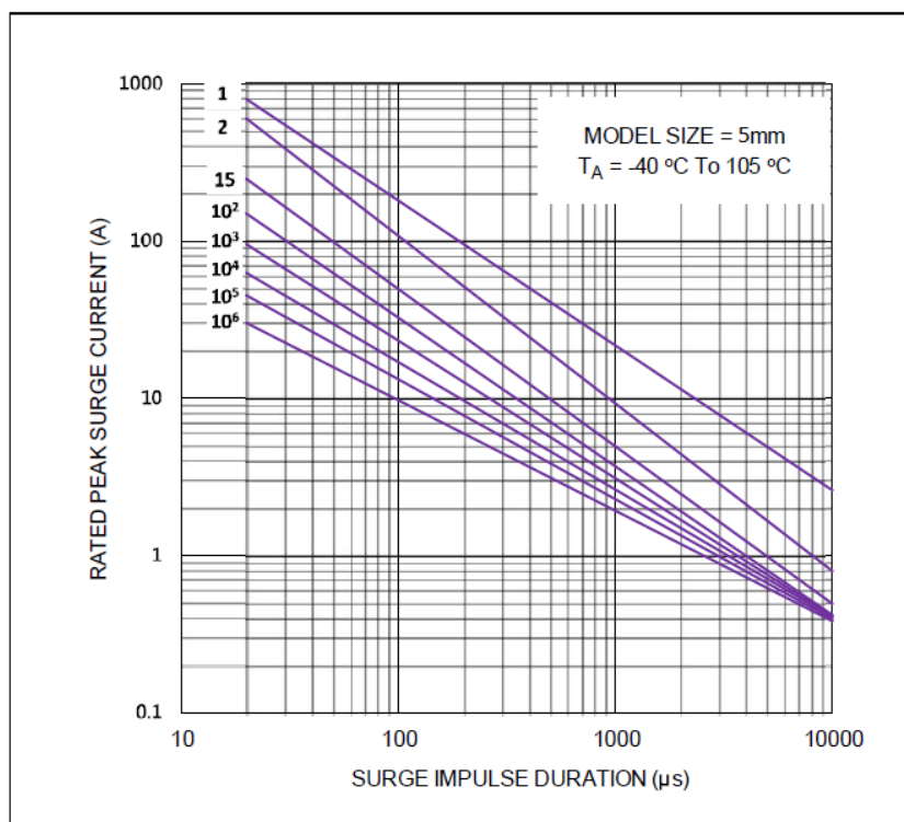
FMOV05201-V to FMOV05751-V
